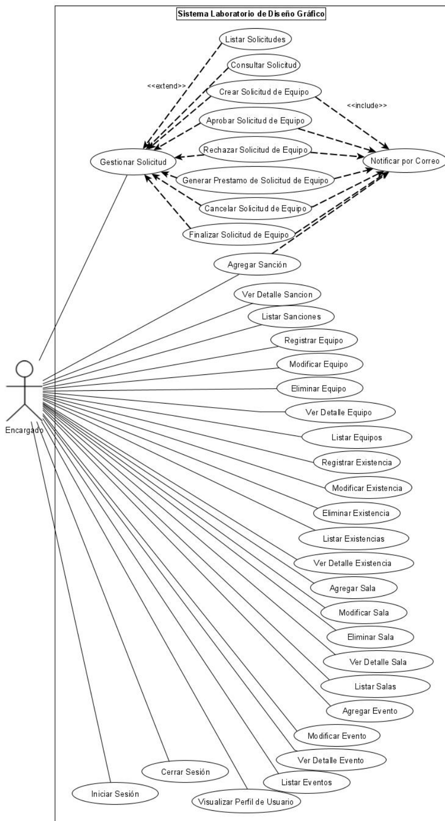
Figura 8: Diagrama de casos de uso de actor encargado.
