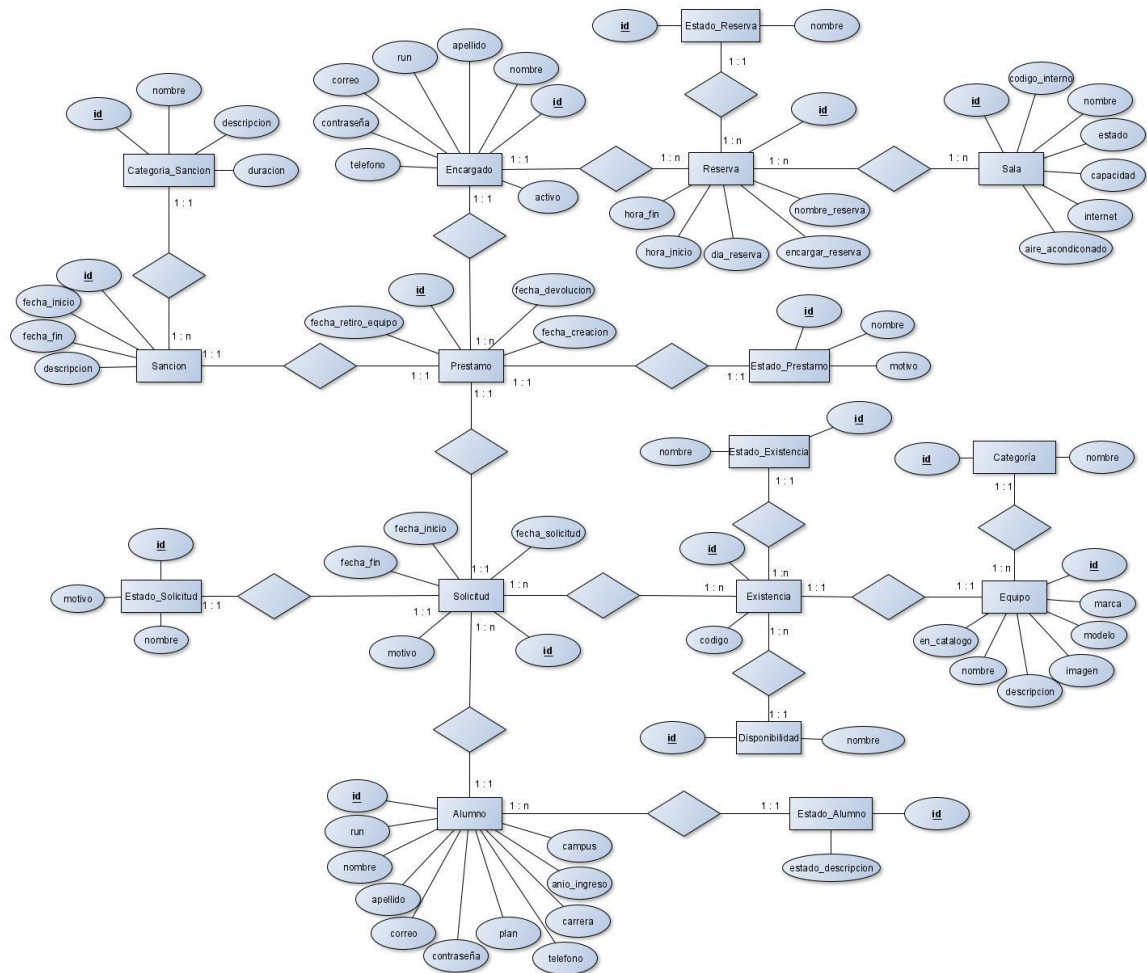
Figura 9: Modelo de Entidad Relación.
