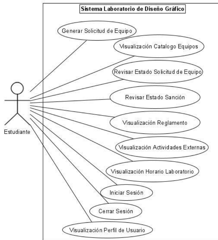
Figura 7: Diagrama de casos de uso del actor estudiante.
