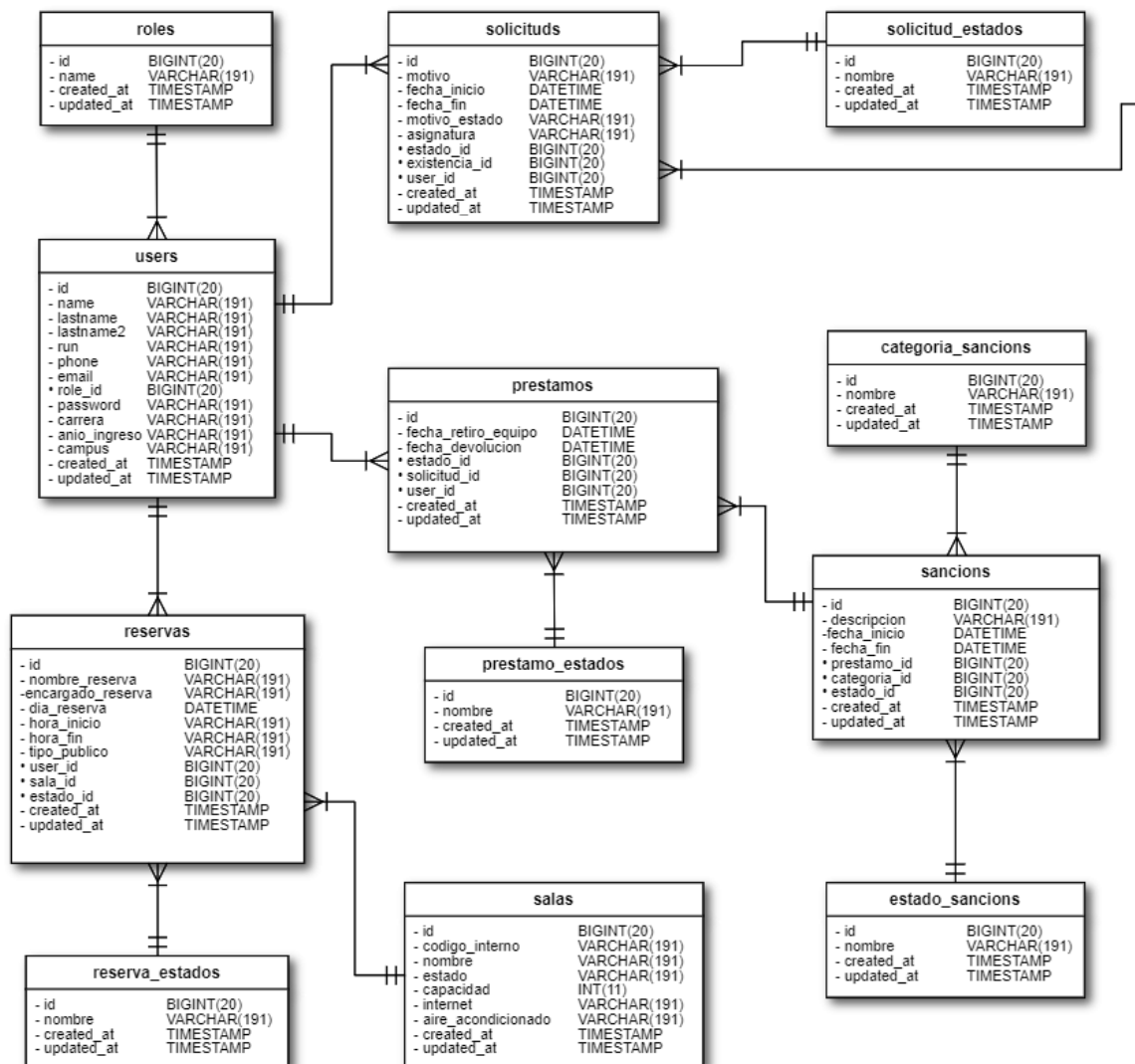
Figura 10: Diseño físico de la Base de datos
