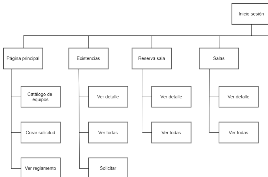
Figura 29: Mapa de navegación perfil alumno.
