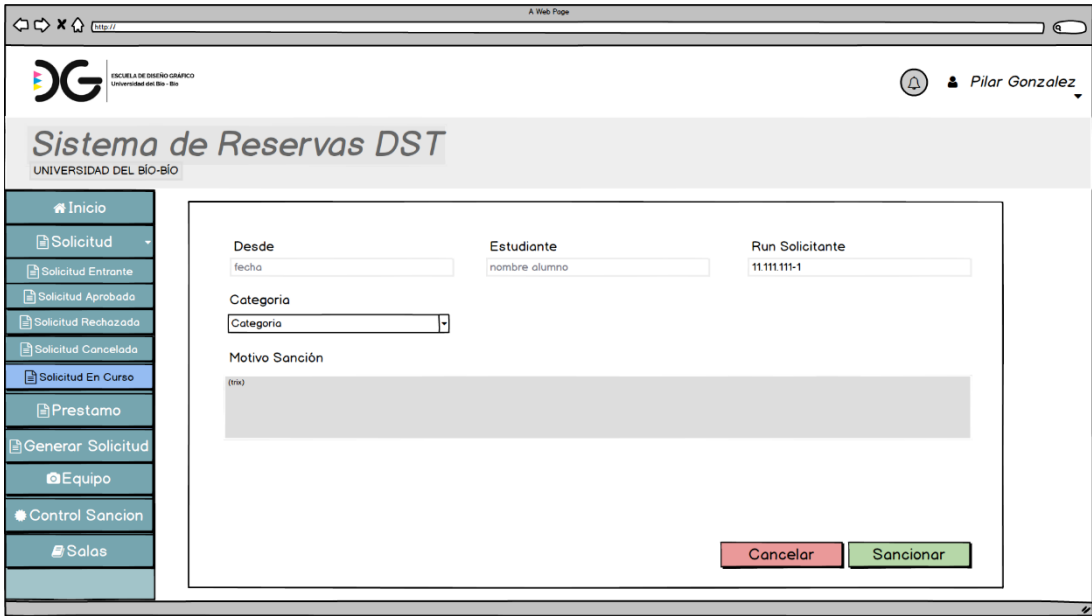
Figura 15: Interfaz de módulo de solicitud en curso con acción de sanción.
