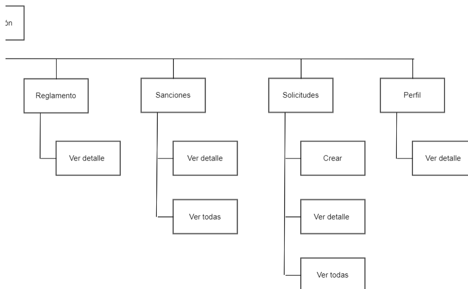
Figura 30: Mapa de navegación perfil alumno (continuación).
