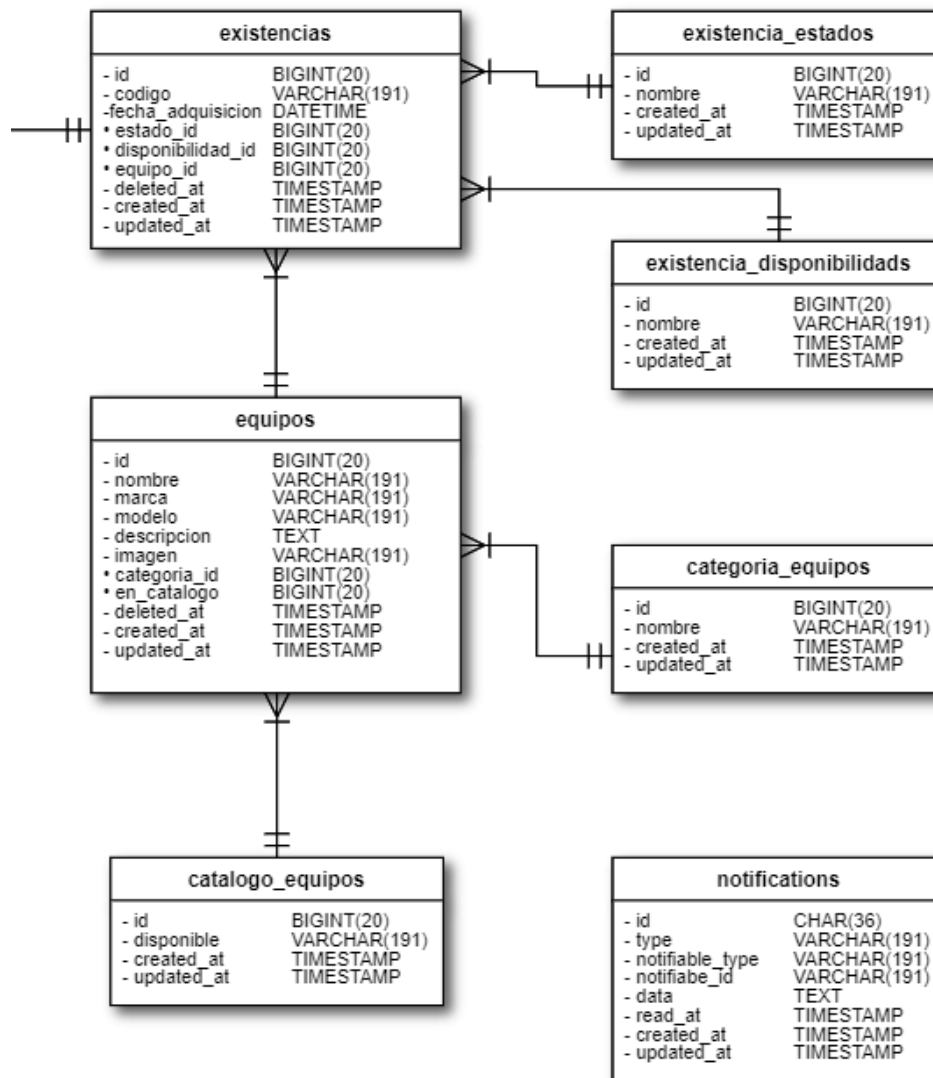
Figura 11: Diseño físico de la Base de datos (continuación).
