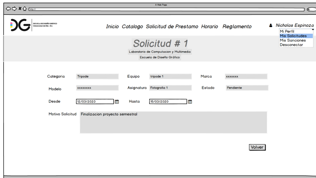
Figura 42: Interfaz módulo: detalle solicitud.
